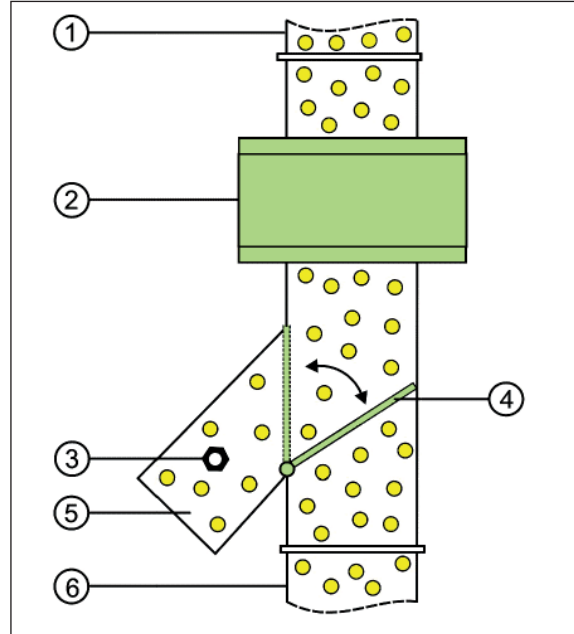
1)Đầu vào 2)Cuộn dò 3)Tạp chất kim loại 4)Bẫy sập 5)Đầu ra tạp chất 6)Đầu ra nguyên liệu
