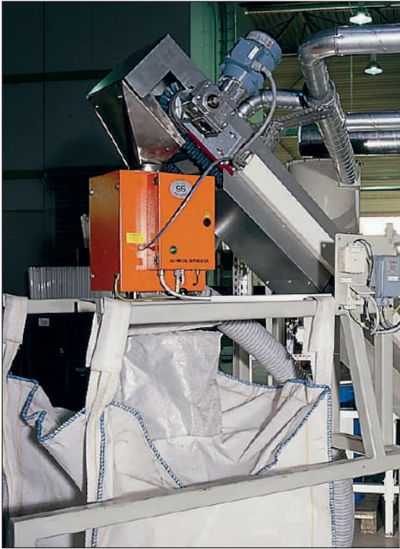
Máy tách kim loại RAPID COMPACT được sử dụng để kiểm tra hàng hóa số lượng lớn trong điều kiện rơi tự do. Thiết bị phát hiện tất cả các tạp chất kim loại từ tính và phi từ tính (thép, thép không gỉ, nhôm) - ngay cả khi tạp chất nằm bên trong sản phẩm. Các tạp chất kim loại được loại bỏ thông qua thiết bị reject "Quick Flap"
