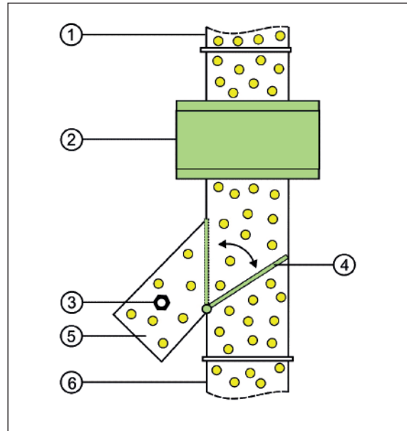
1) Cửa nạp liệu 2) Cuộn dò 3) Tạp chất kim loại 4) Nắp tách 5) Nguyên liệu bị loại bỏ 6) Nguyên liệu tốt
